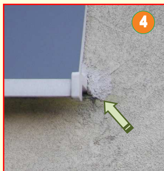
dodatočne vymieňaný parapetný plech
