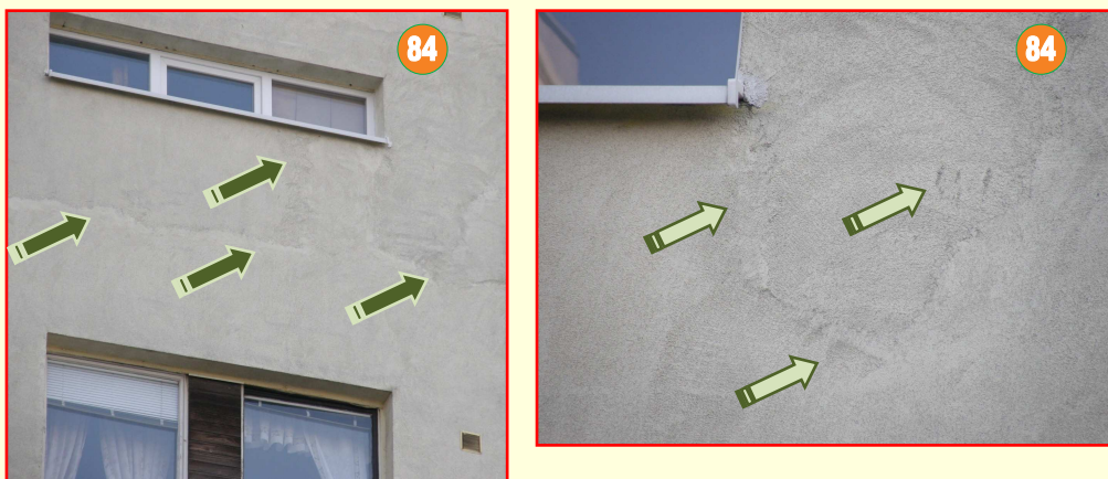
nekvalitne vykonaná vrchná povrchová vrstva
