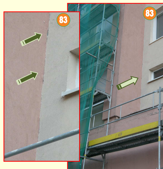
styk obvodového plášťa a schodiska
