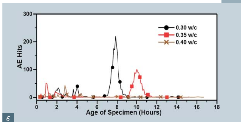
Obr. 5 Korelácia intenzity akustickej emisie čerstvého betónu a začiatku tuhnutia [15]
